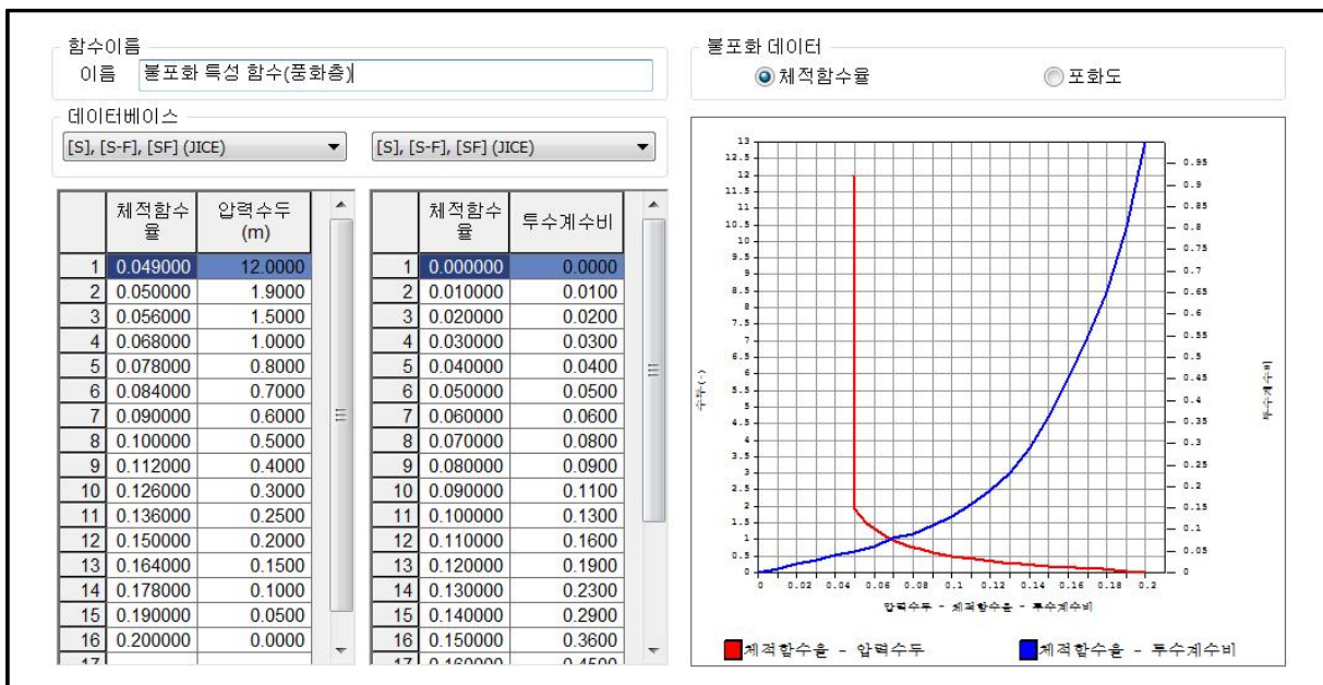
【그림 47.15】 압력수두-체적함수물(포화도)-투수계수비 함수
