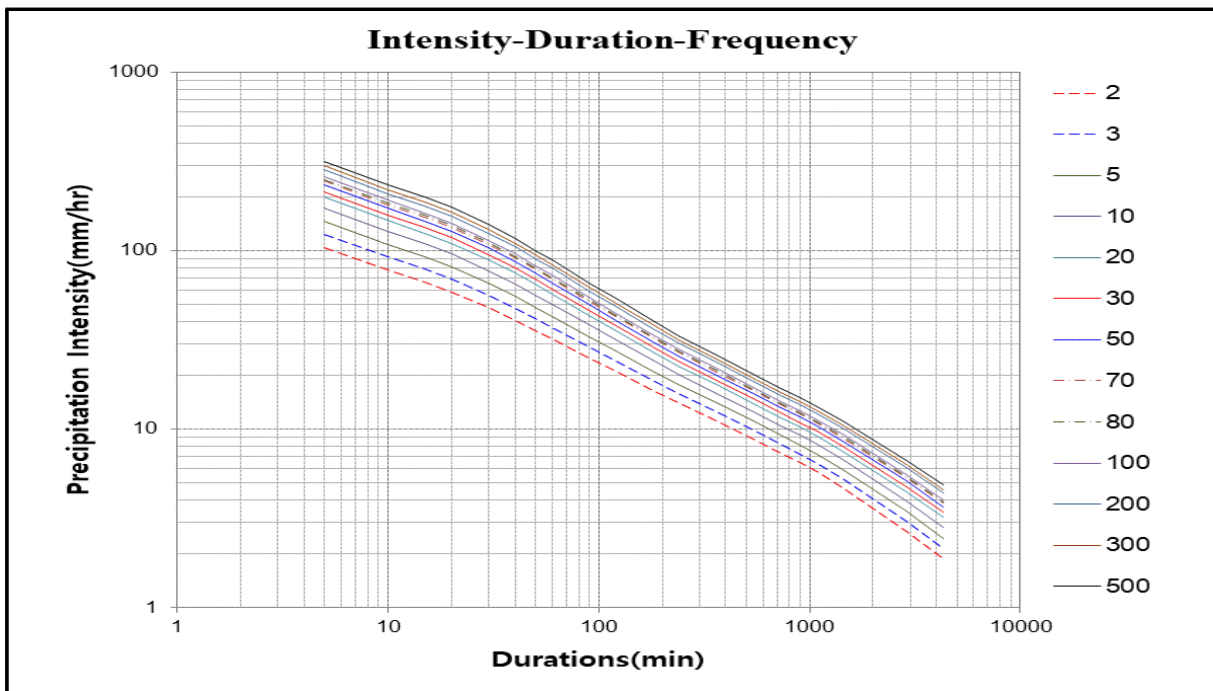
【그림 47.9】 영천지역 IDF곡선
