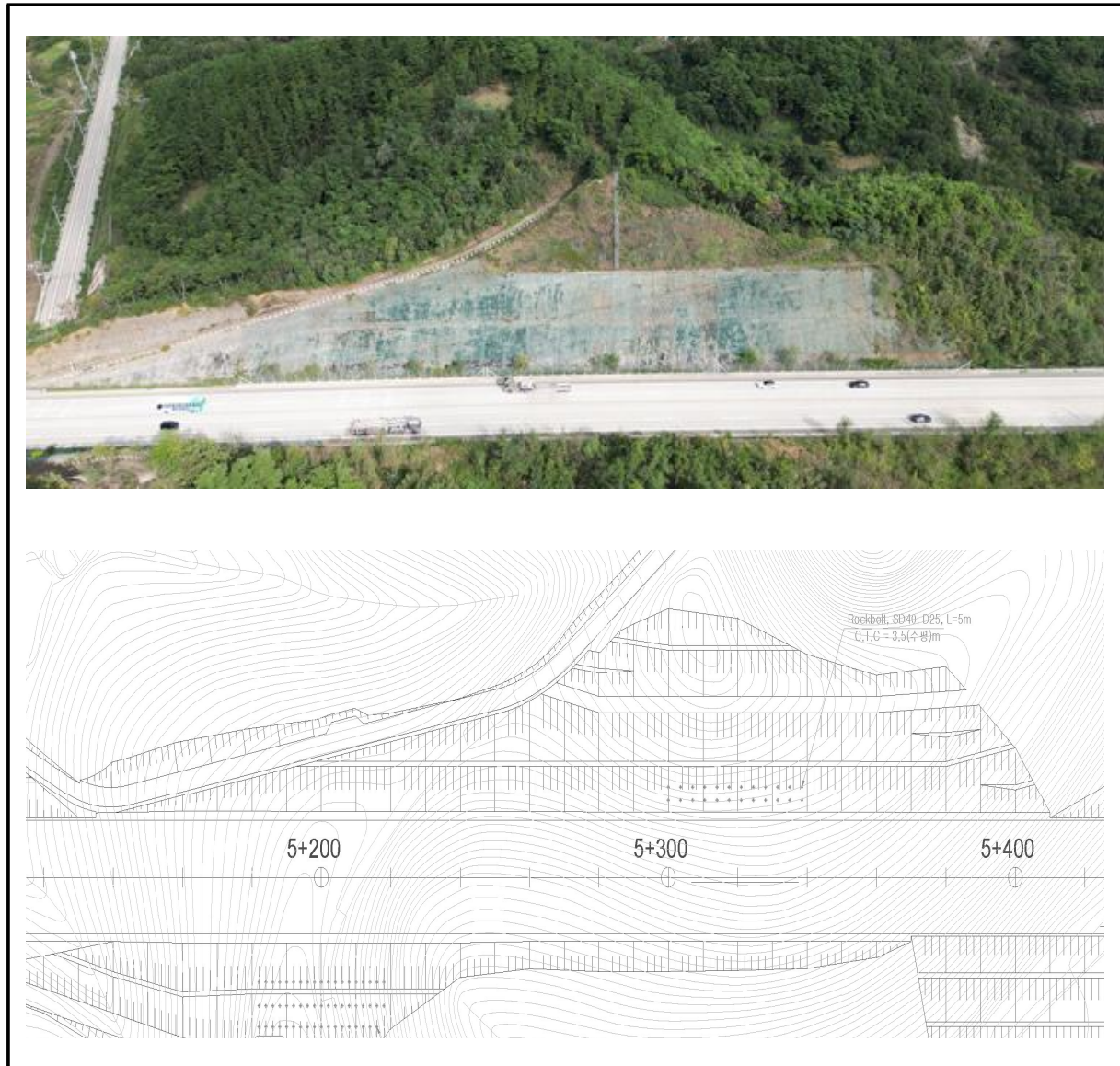
【그림 47.14】 상주절토47 검토대상 비탈면구간
